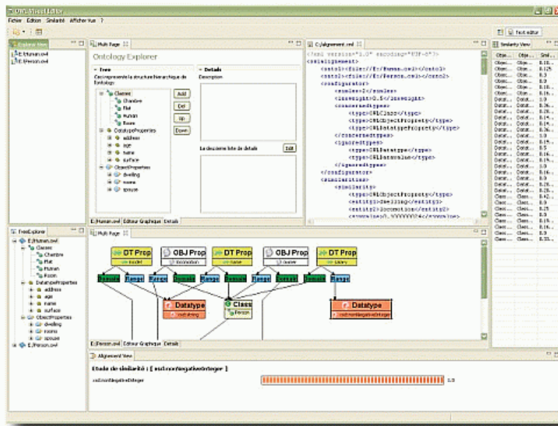
Fig. 4. Un editor visuale di OWL.
